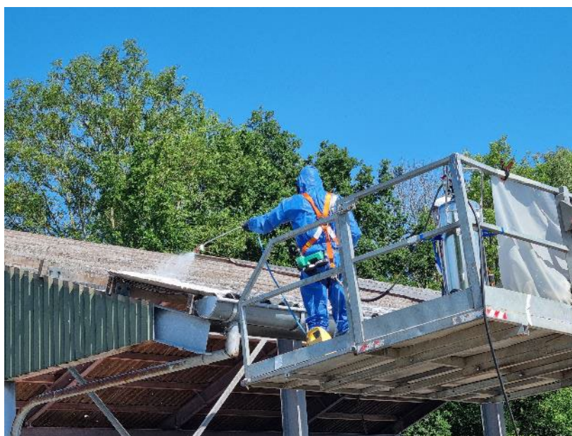
Foto 22: Inschuimen asbestdak vanuit verreiker
